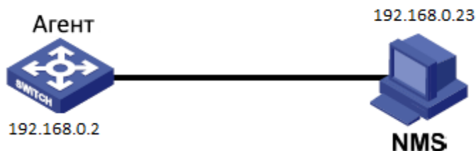
Рис. 112. Пример настройки SNMPv2
