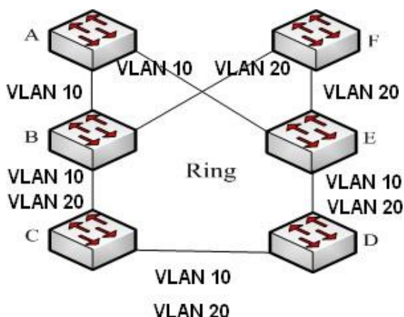
Рис. 206. Sy2-VLAN-Ring
