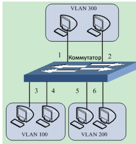
Рис. 198. Пример настройки PVLAN
