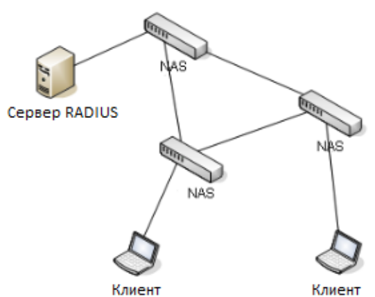
Рис. 134. Структура RADIUS
