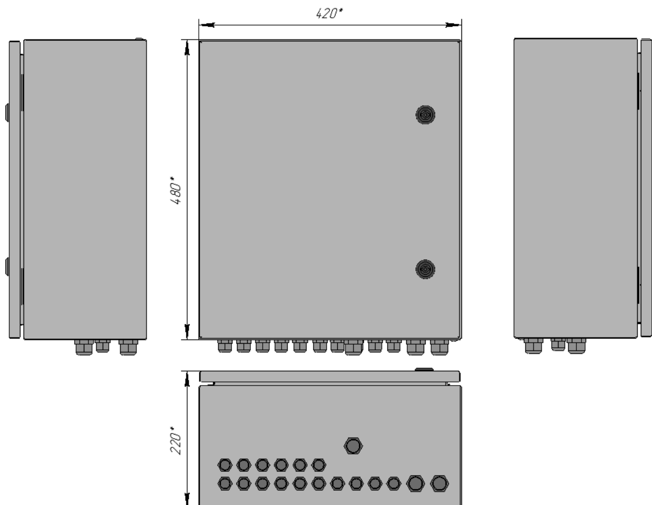
Рисунок 1 Внешний вид и габаритные размеры Узла доступа 0168S2-F
