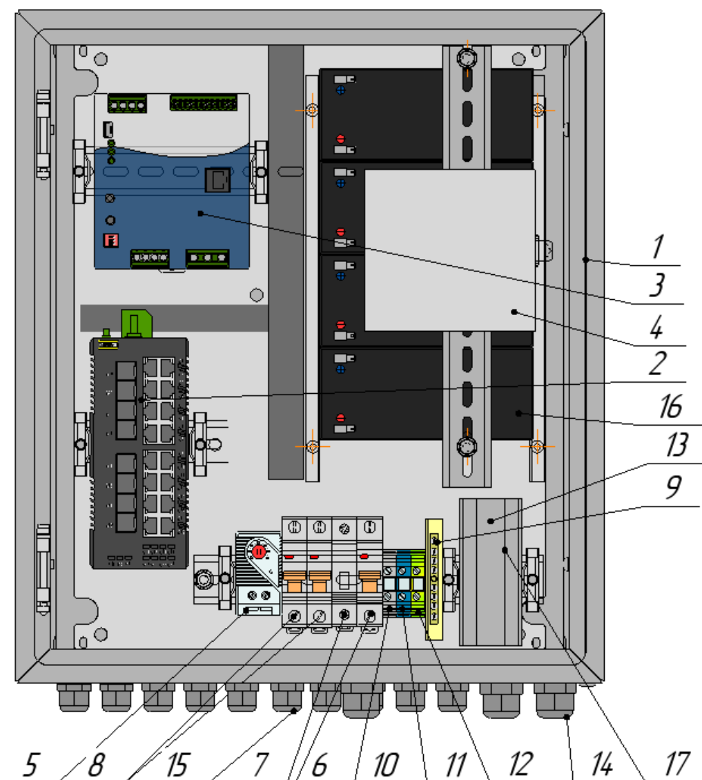
Рисунок 2. Схема расположения оборудования Узла доступа 0168S2-F
