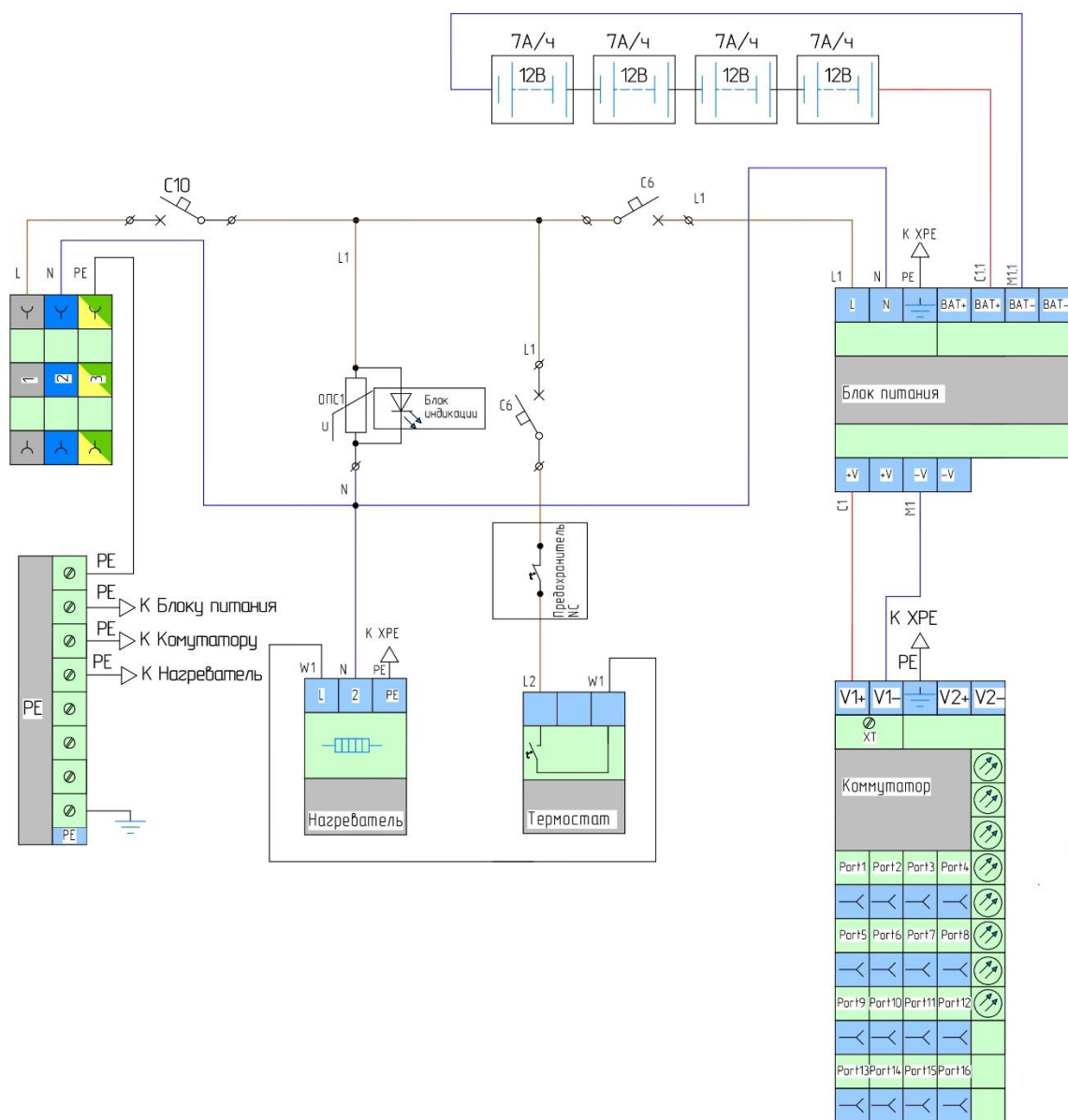
Рисунок 3. Электрическая схема Узла доступа 0168S2-F
