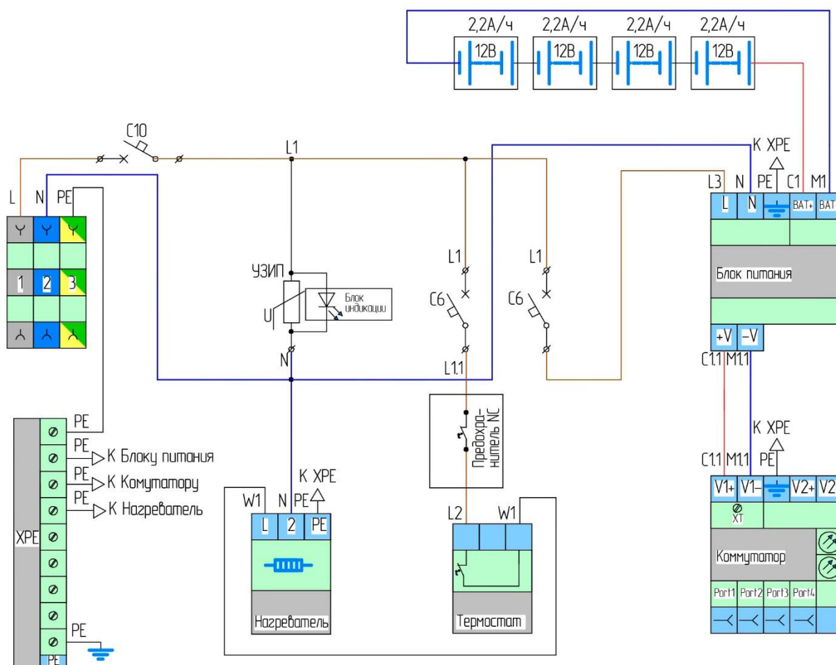
Рисунок 3. Электрическая схема Узла доступа 042S2-F
