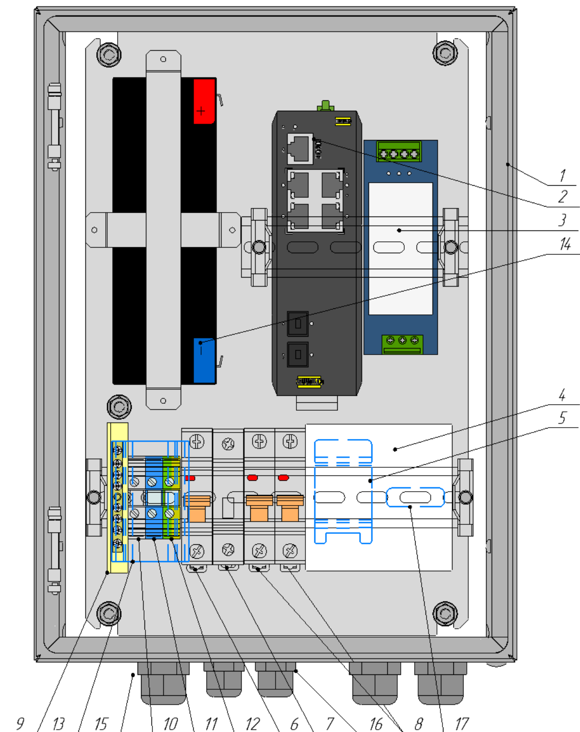
Рисунок 2. Схема расположения оборудования Узла доступа 042S2-F
