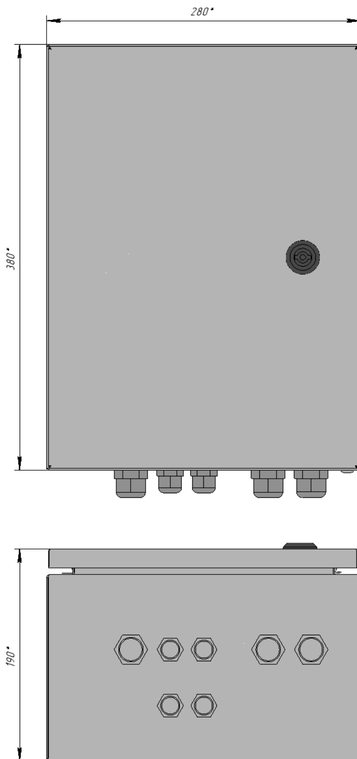
Рисунок 1 Внешний вид и габаритные размеры Узла доступа 042S2-F
