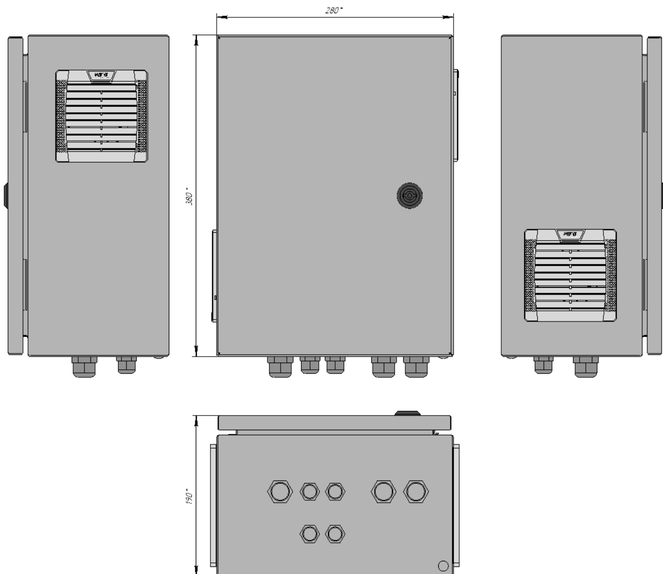
Рисунок 1 Внешний вид и габаритные размеры Узла доступа 042S3-F
