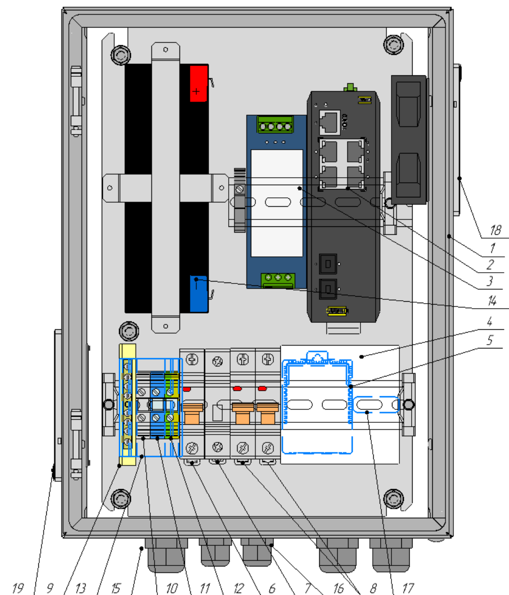
Рисунок 2. Схема расположения оборудования Узла доступа 042S3-F
