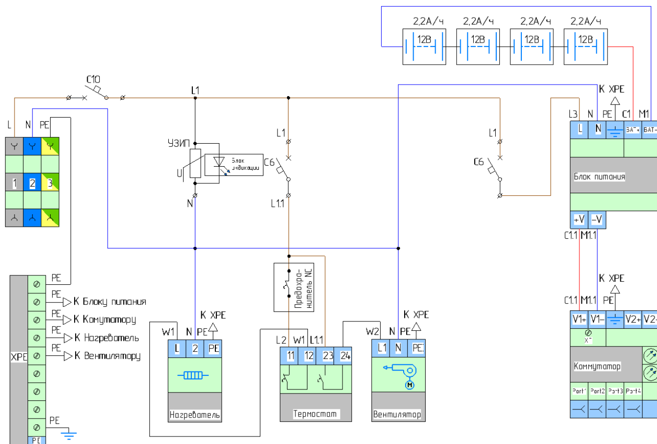
Рисунок 3. Электрическая схема Узла доступа 042S3-F
