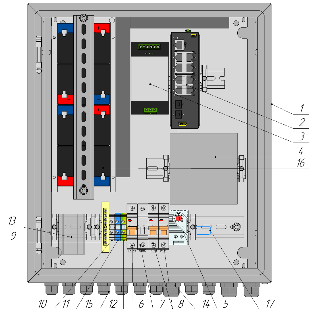
Рисунок 2. Схема расположения оборудования Узла доступа 082S2-F
