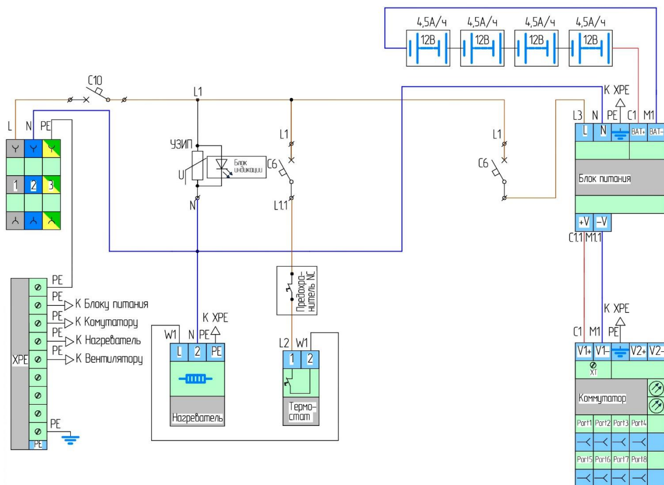
Рисунок 3. Электрическая схема Узла доступа 082S2-F
