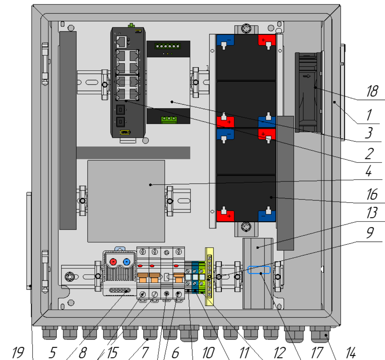
Рисунок 2. Схема расположения оборудования Узла доступа 082S3-F
