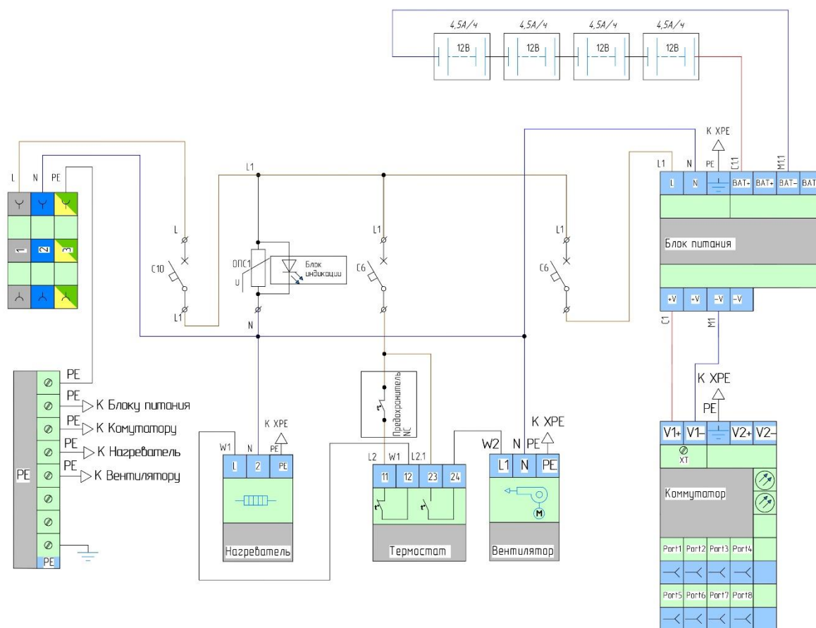
Рисунок 3. Электрическая схема Узла доступа 082S3-F
