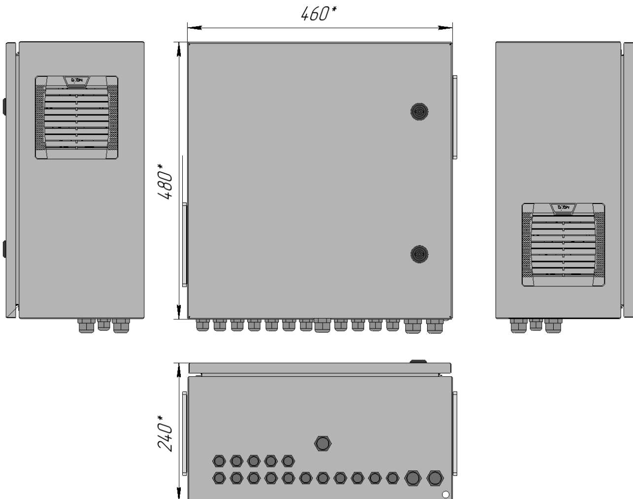
Рисунок 1 Внешний вид и габаритные размеры Узла доступа 082S3-F
