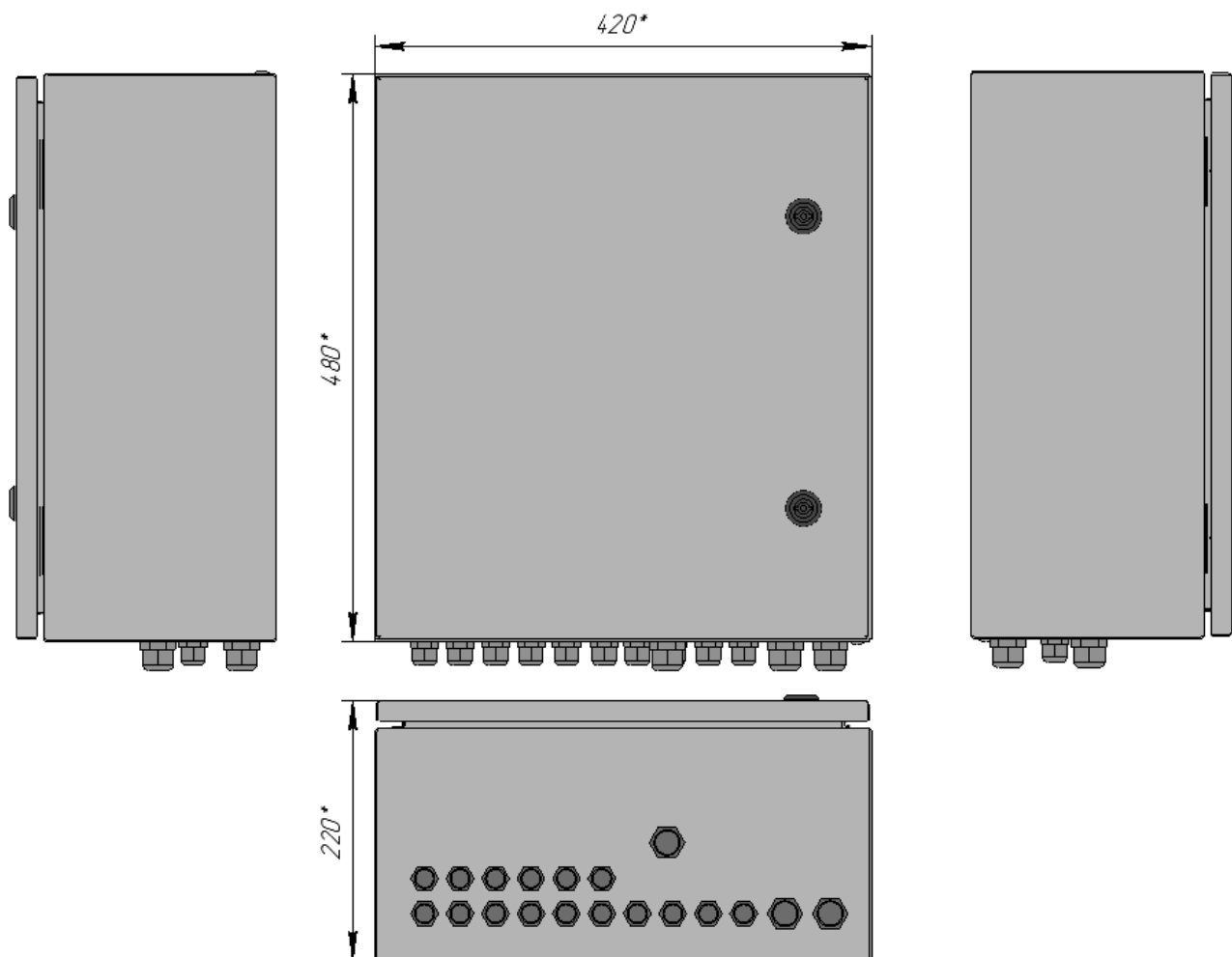
Рисунок 1 Внешний вид и габаритные размеры Узла доступа 1158S2-F
