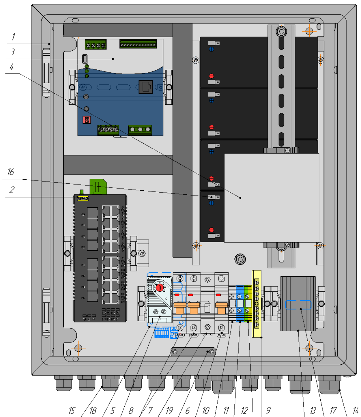
Рисунок 2. Схема расположения оборудования Узла доступа 1158S2-F
