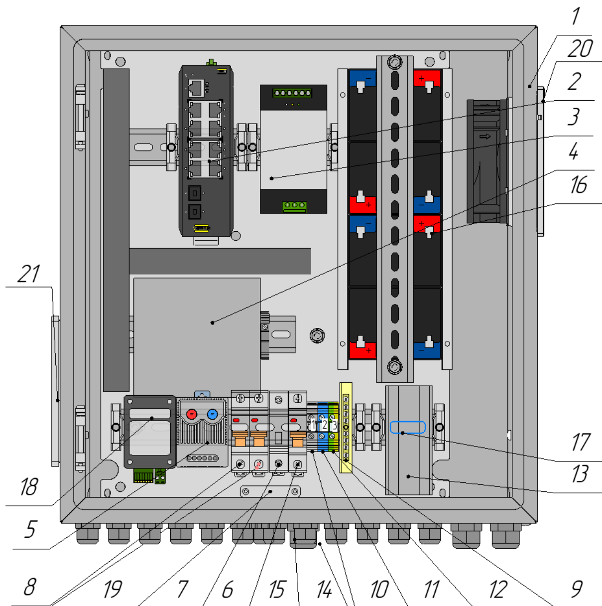
Рисунок 3. Схема расположения оборудования Узла доступа 172S3-F
