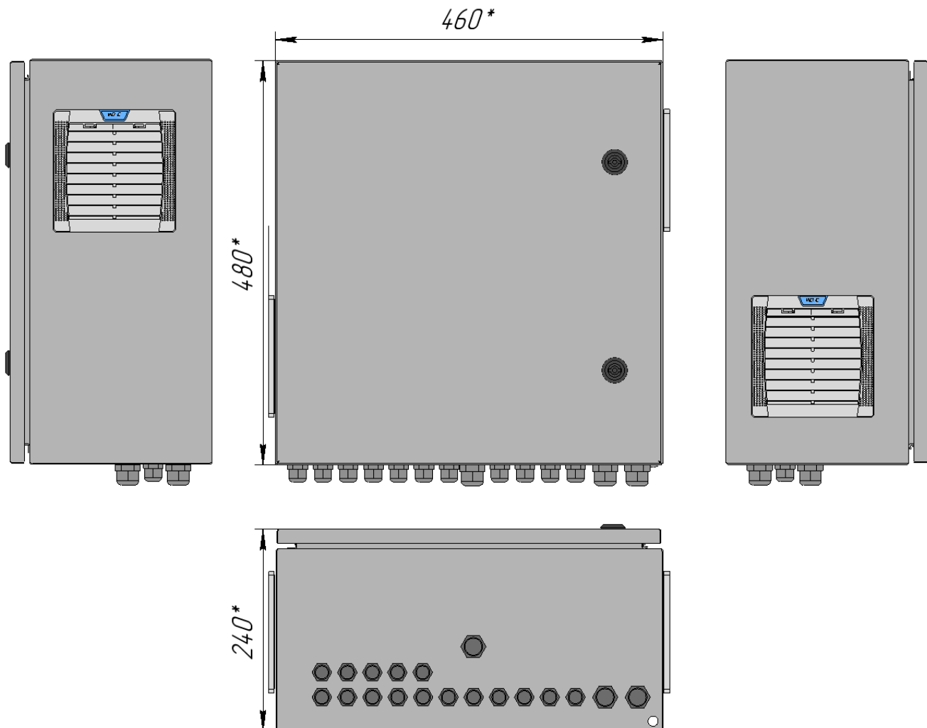
Рисунок 1 Внешний вид и габаритные размеры Узла доступа 172S3-F
