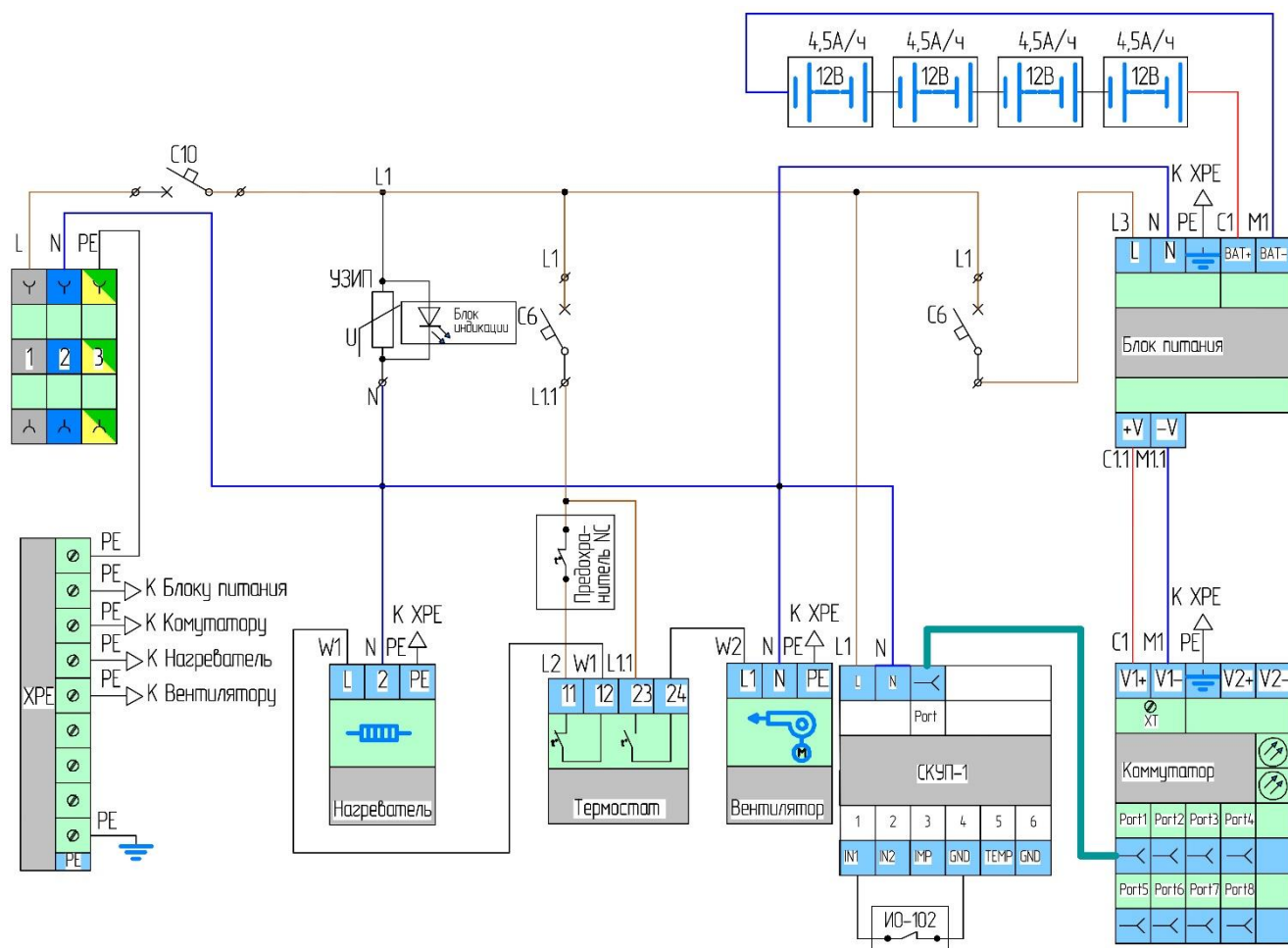
Рисунок 3. Электрическая схема Узла доступа 172S3-F
