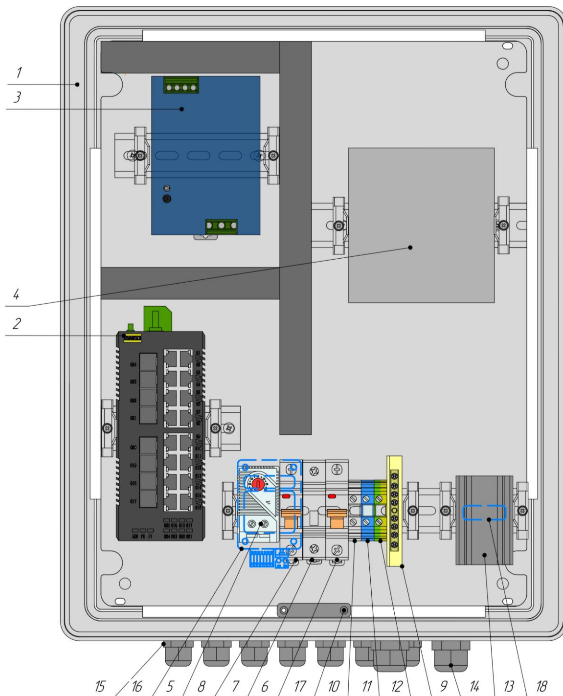
Рисунок 3. Схема расположения оборудования Узла доступа 1158S1-PL
