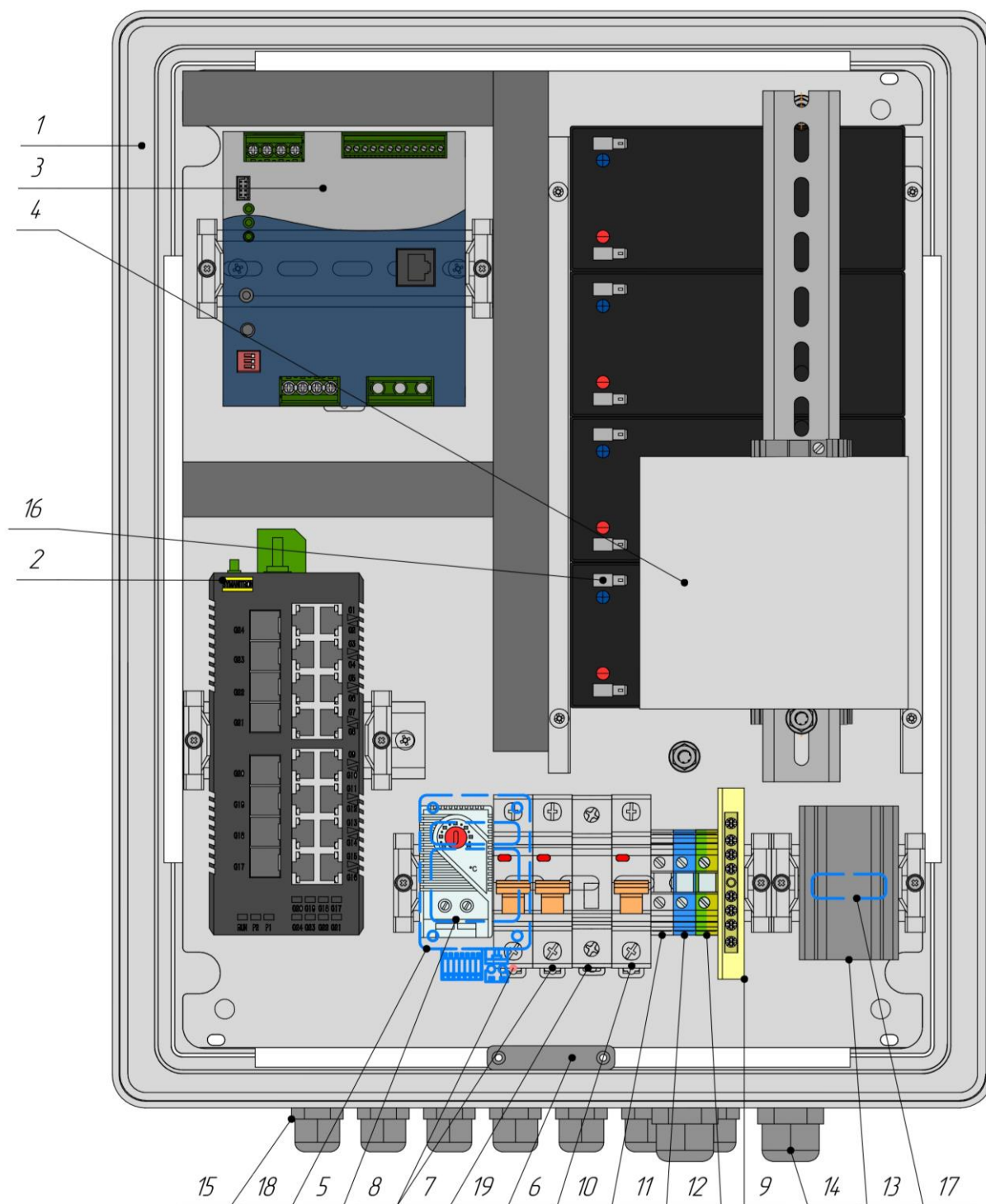
Рисунок 3. Схема расположения оборудования Узла доступа 1158S2-PL
