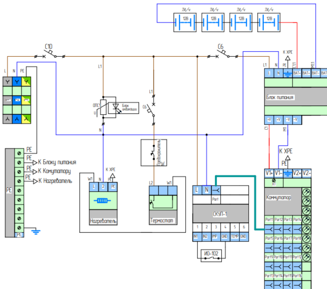
Рисунок 2. Электрическая схема Узла доступа 1158S2-PL
