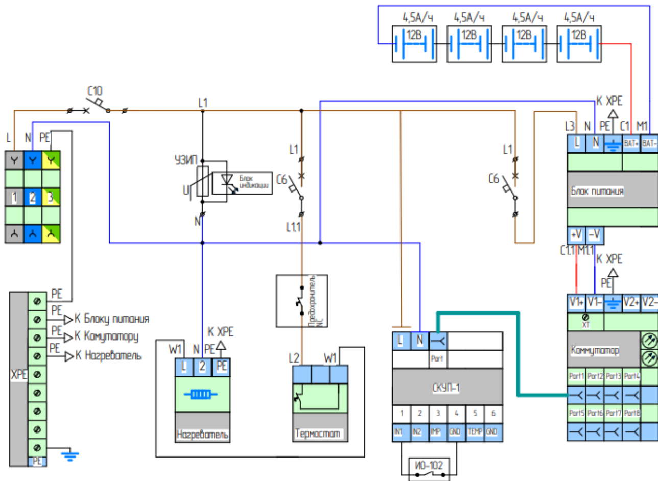
Рисунок 2. Электрическая схема Узла доступа 172S2-PL
