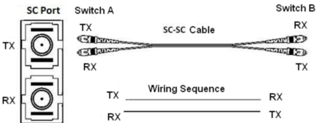
Рис. 100Base-FX порт подключения
