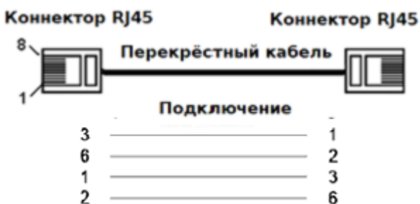
Рис. Подключения перекрытого кабеля
