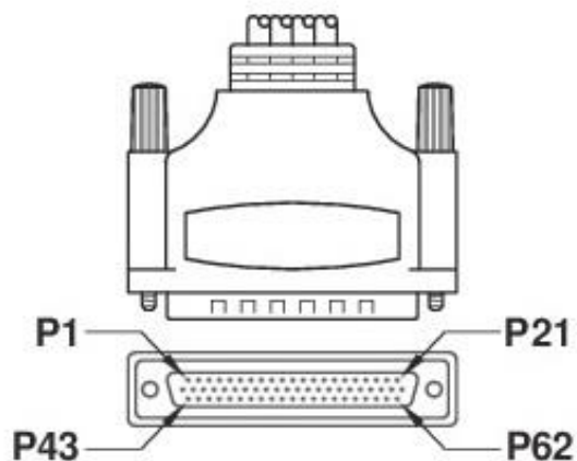
Вилка DB62 с 4 портами RS-232
