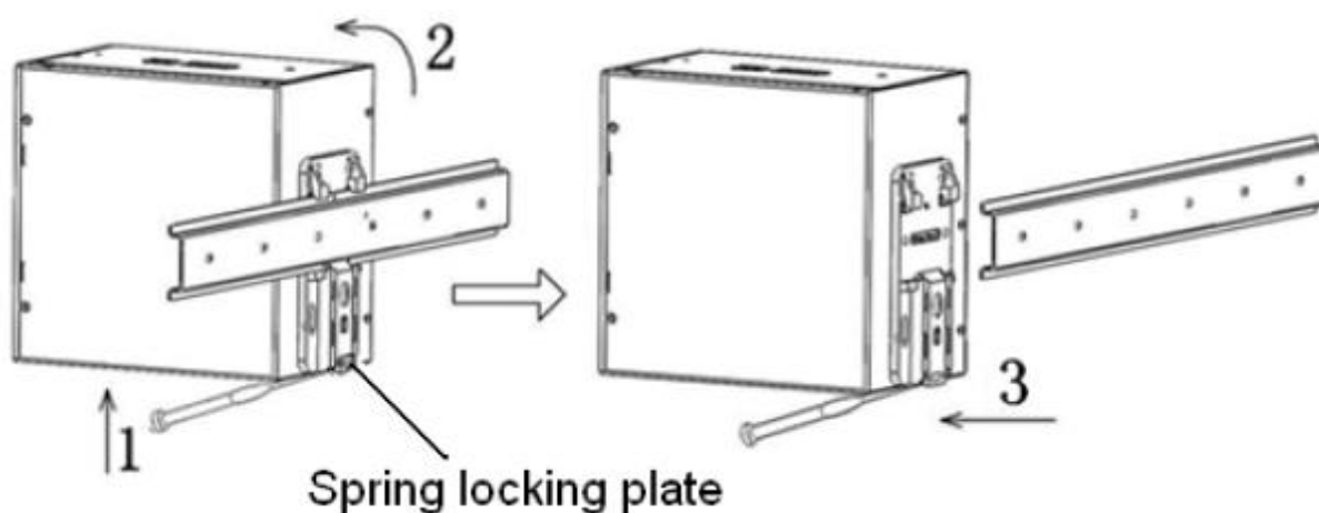
Рис. Снятие с DIN-рейки
