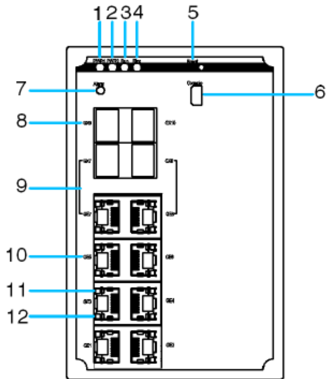
Рис. Передняя панель SEWMG10-D -2GSFP2GT - 2GSFP -6GT
