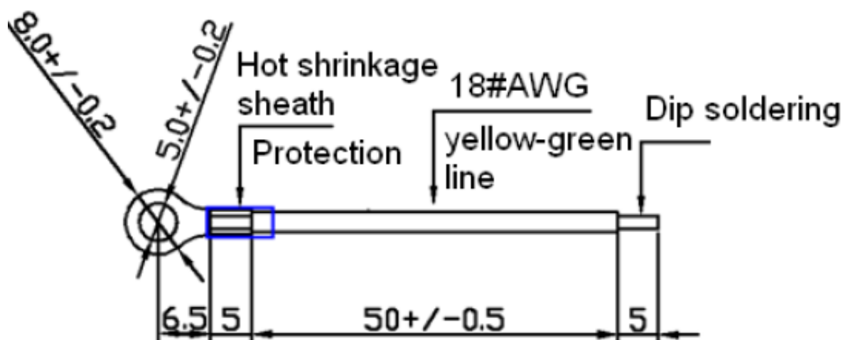
Рис. Размеры кабеля заземления
