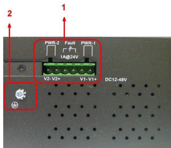
Рис. 4 Верхняя панель
