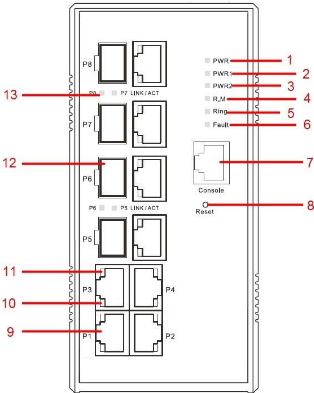
Рис.3 Передняя панель
