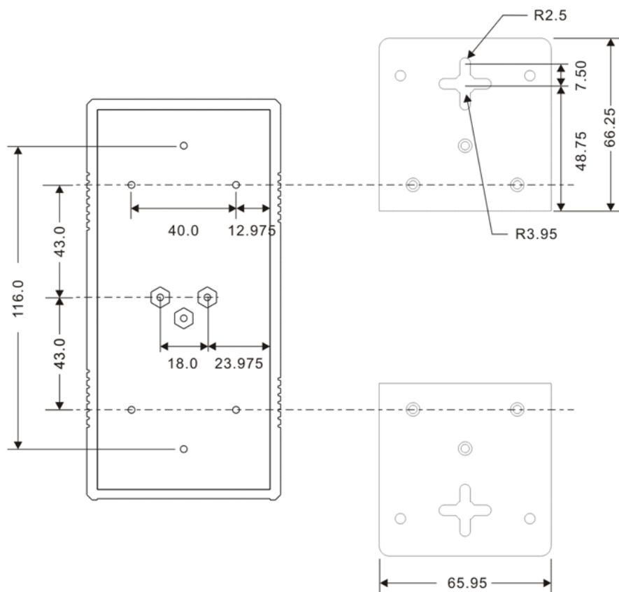
Рис.2 Размеры настенного крепления
