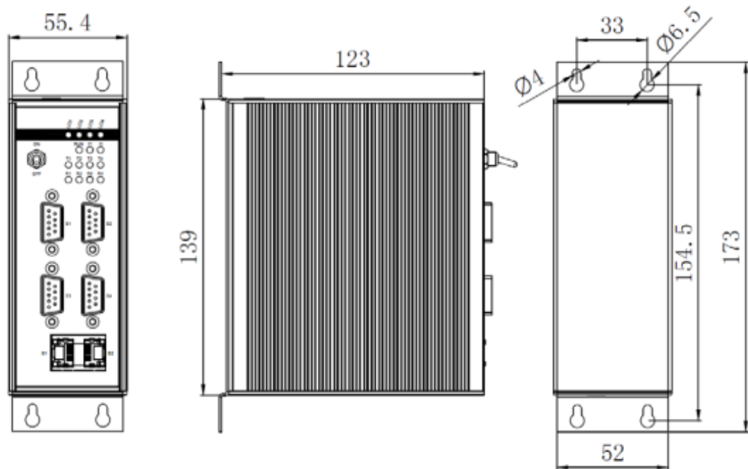
Рис. Размеры устройства для монтажа на панель
