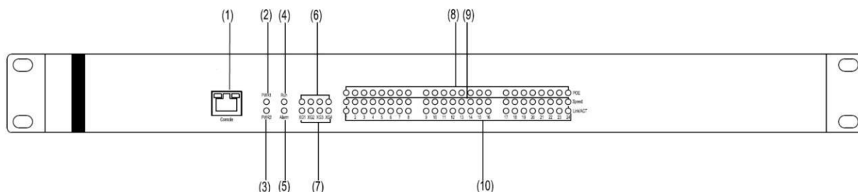
Рисунок 1 – Передняя панель
