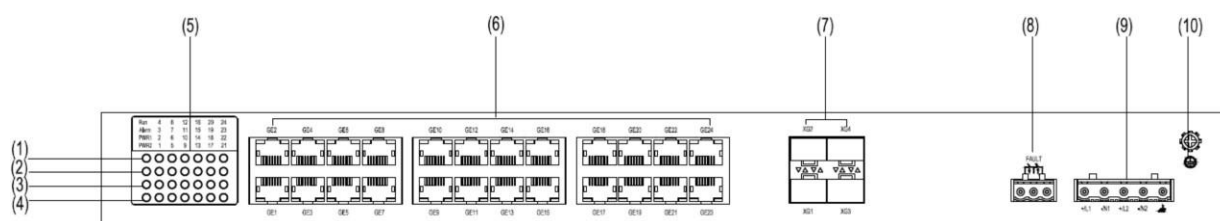
Рисунок 2 – Задняя панель
