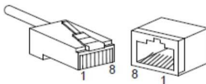
Рисунок 5 – Разъем RJ45
