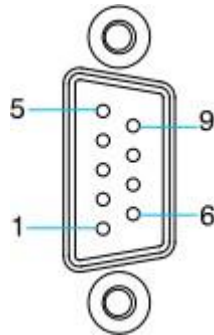
Рис. Разъём DB9
