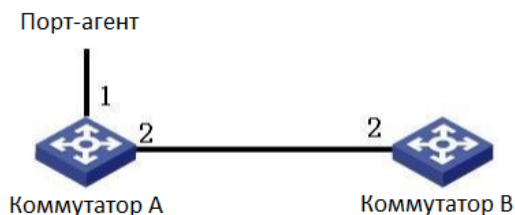
Рис. 184. Сеть GMRP
