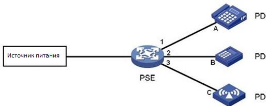
Рис. 188. Система питания PoE
