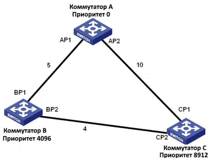
Рис. 231. Пример настройки RSTP
