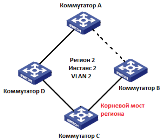
Рис. 236. Сопоставление VLAN 2 к Инстансу 2
