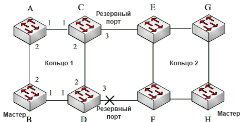
Рис. 212. Топология Sy2-Ring+
