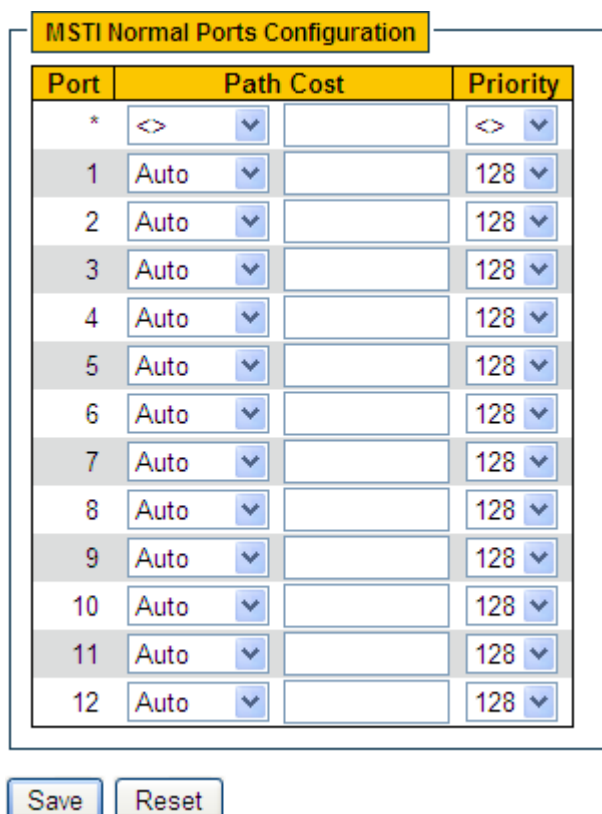
Рис. 243. Настройка портов MSTI
