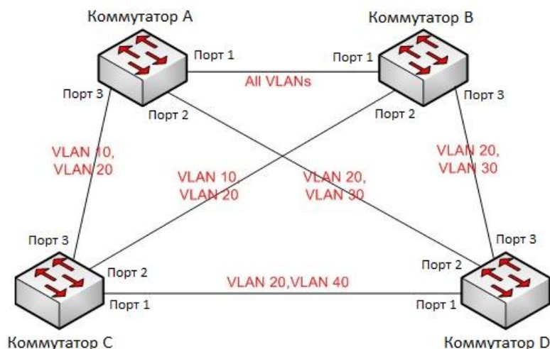
Рис. 247. Пример типовой настройки MSTP
