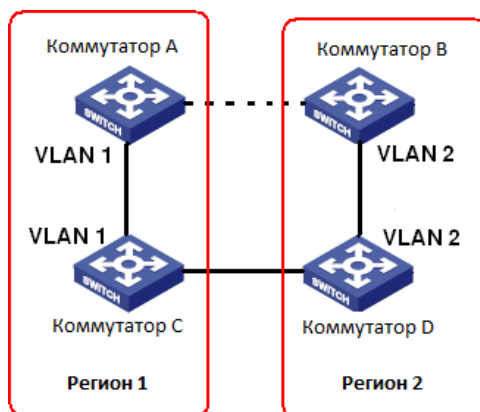
Рис. 233. Топология MSTP
