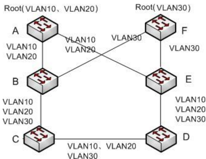
Рис. 219. Sy2-RP-VLAN-Based
