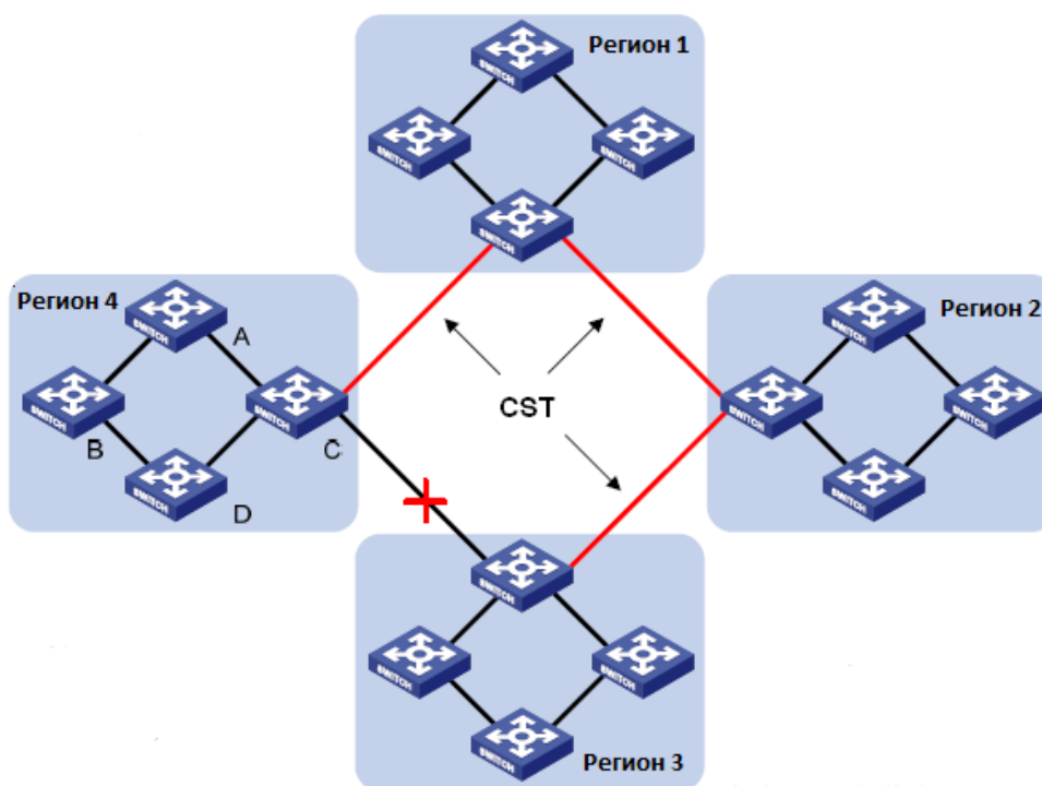
Рис. 234. Концепция MSTP
