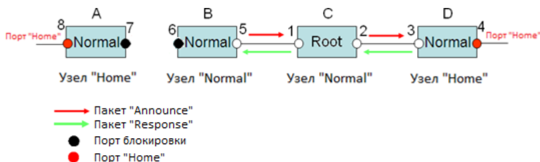
Рис. 223. Восстановление связи с Dual Homing
