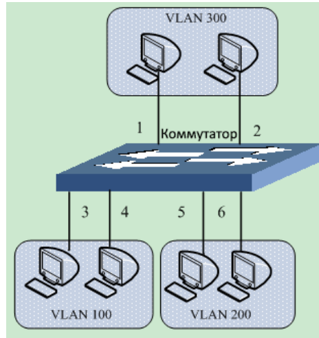
Рис. 203. Пример настройки PVLAN
