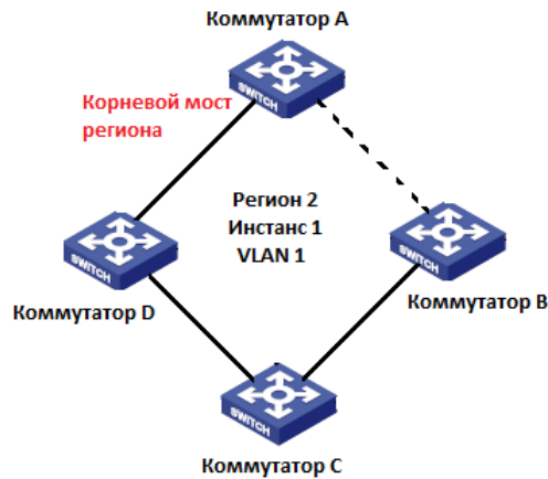
Рис. 235. Сопоставление VLAN 1 к Инстансу 1
