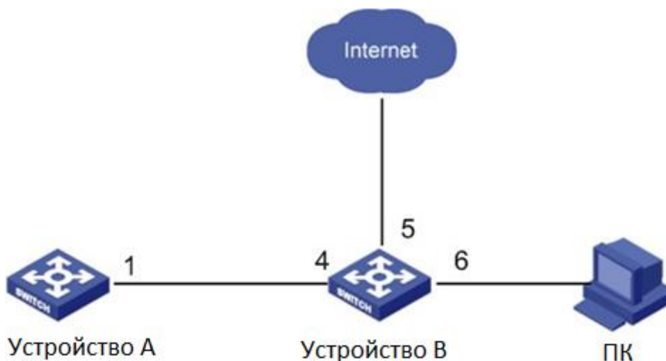
Рис. 208. Пример настройки GVRP
