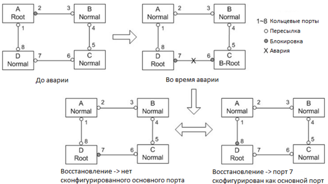
Рис. 218. Восстановление сети с Sy2-RP
