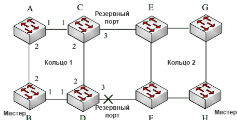
Рис. 220. Резервирование Sy2-RP
