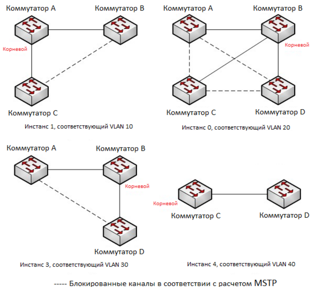
Рис. 248. Инстансы связующего дерева для каждой VLAN
