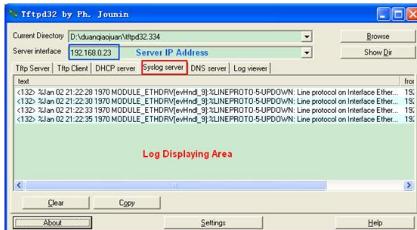
Рис. 260. Загрузка информации системного журнала на сервер в реальном времени
