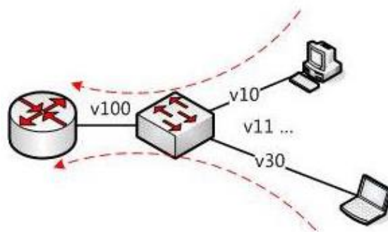
Рис. 138. Схема PVLAN
