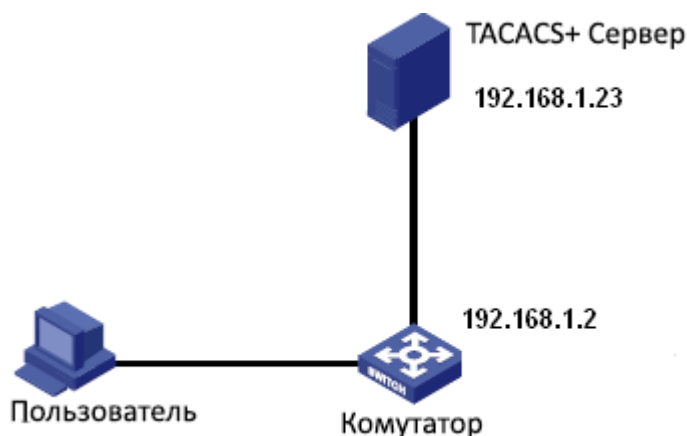
Рис. 130. Пример аутентификации TACACS+
