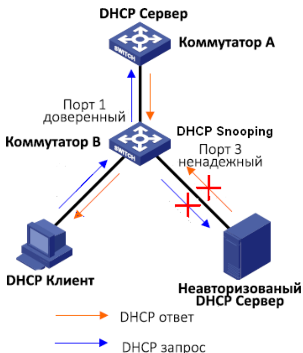
Рис. 186. Пример типовой настройки DHCP Snooping
