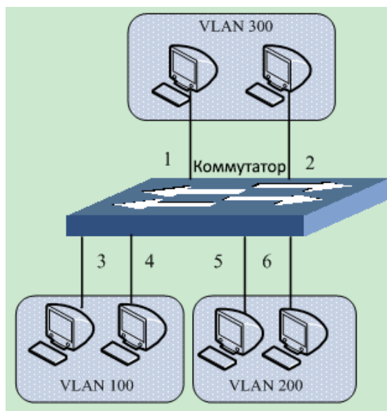
Рис. 141. Пример конфигурации P VLAN
