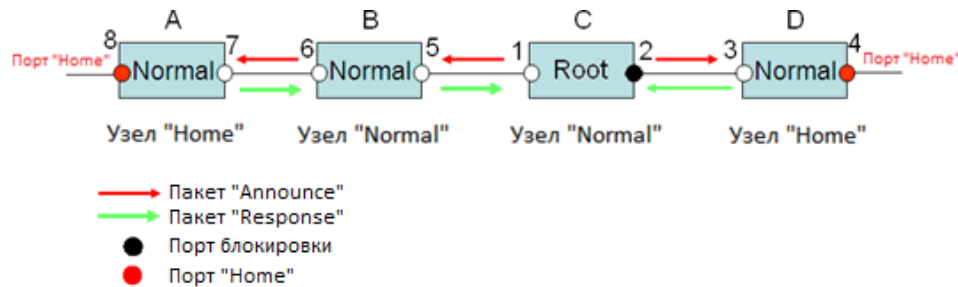
Рис. 70. Конфигурация Dual Homing
