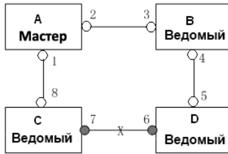
Рис. 51. Восстановление Sy2-Ring
