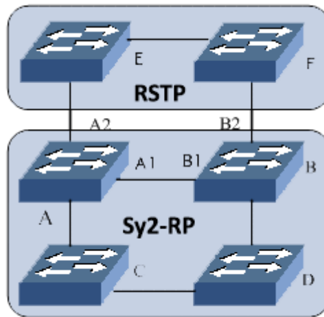
Рис. 63. Применение режима прозрачной передачи RSTP
