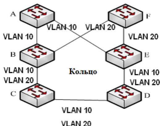
Рис. 53. Sy2-VLAN-Ring
