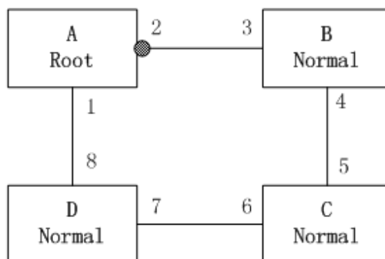
Рис. 65. Топология Sy2-RP
