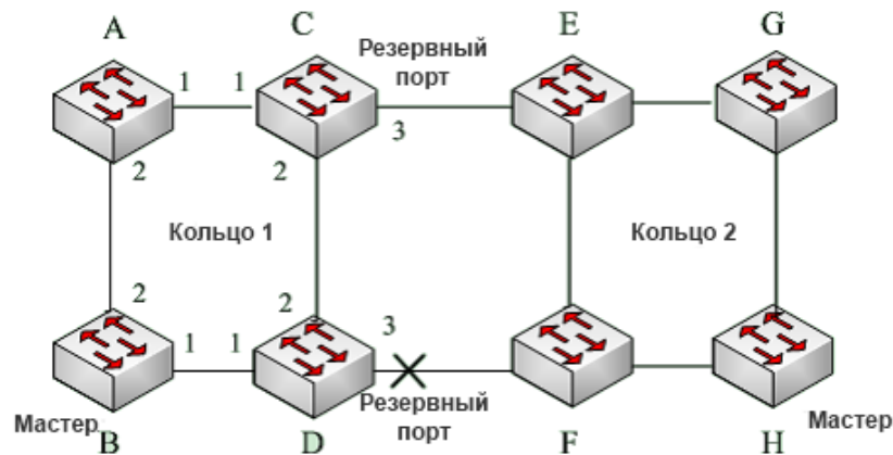
Рис. 52. Топология Sy2-Ring+
