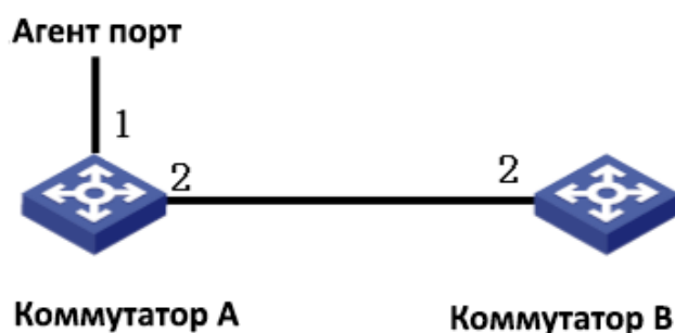
Рис. 81. Сеть GMRP
