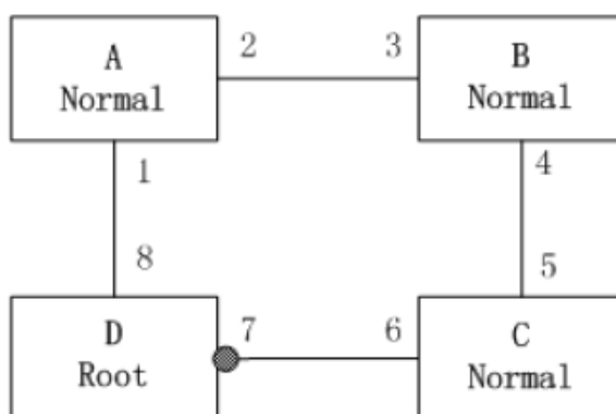
Рис. 67. Восстановление связи
