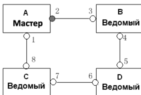
Рис. 50. Топология Sy2-Ring
