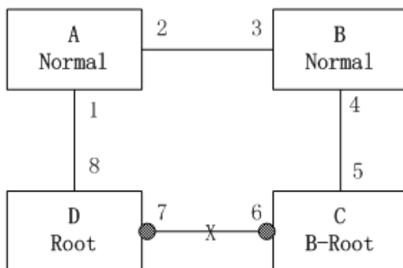
Рис. 66. Обрыв связи
