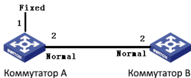
Рис. 145. Пример настройки GVRP
