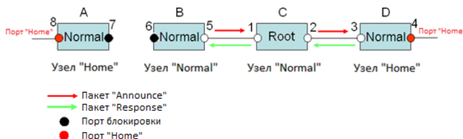
Рис. 71. Восстановление связи Dual Homing
