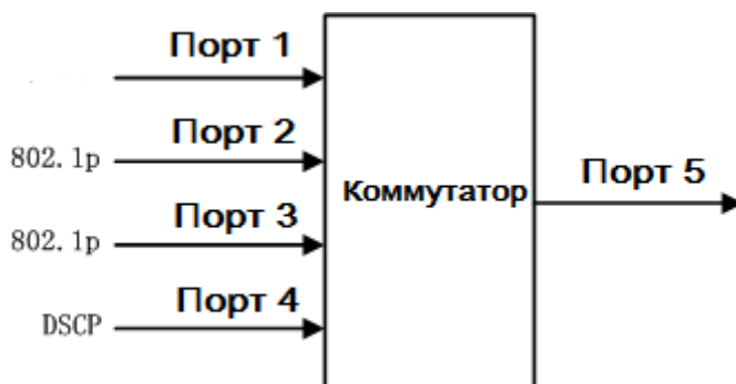
Рис. 41. Пример настройки QoS
