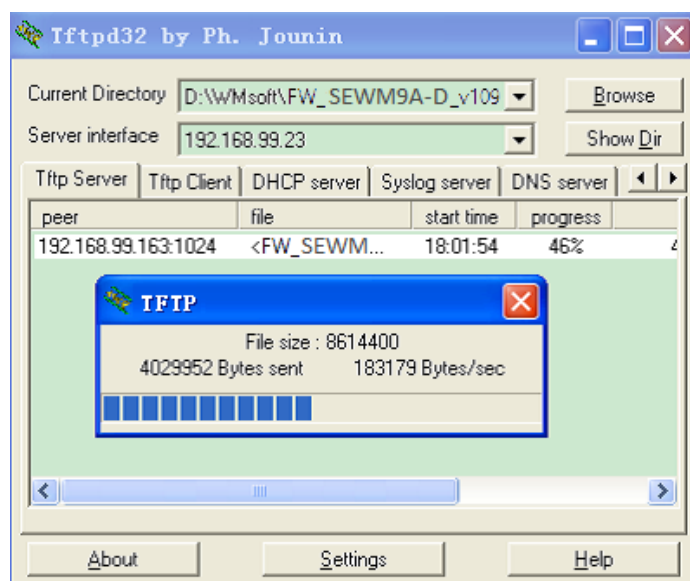
Рис. 26. Соединение коммутатора и сервера TFTP
