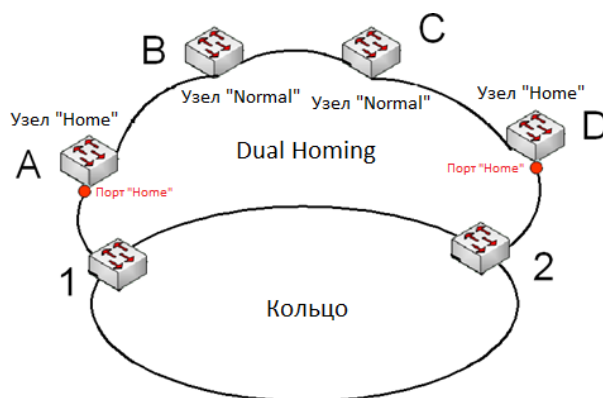
Рис. 69. Реализация протокола Dual Homing
