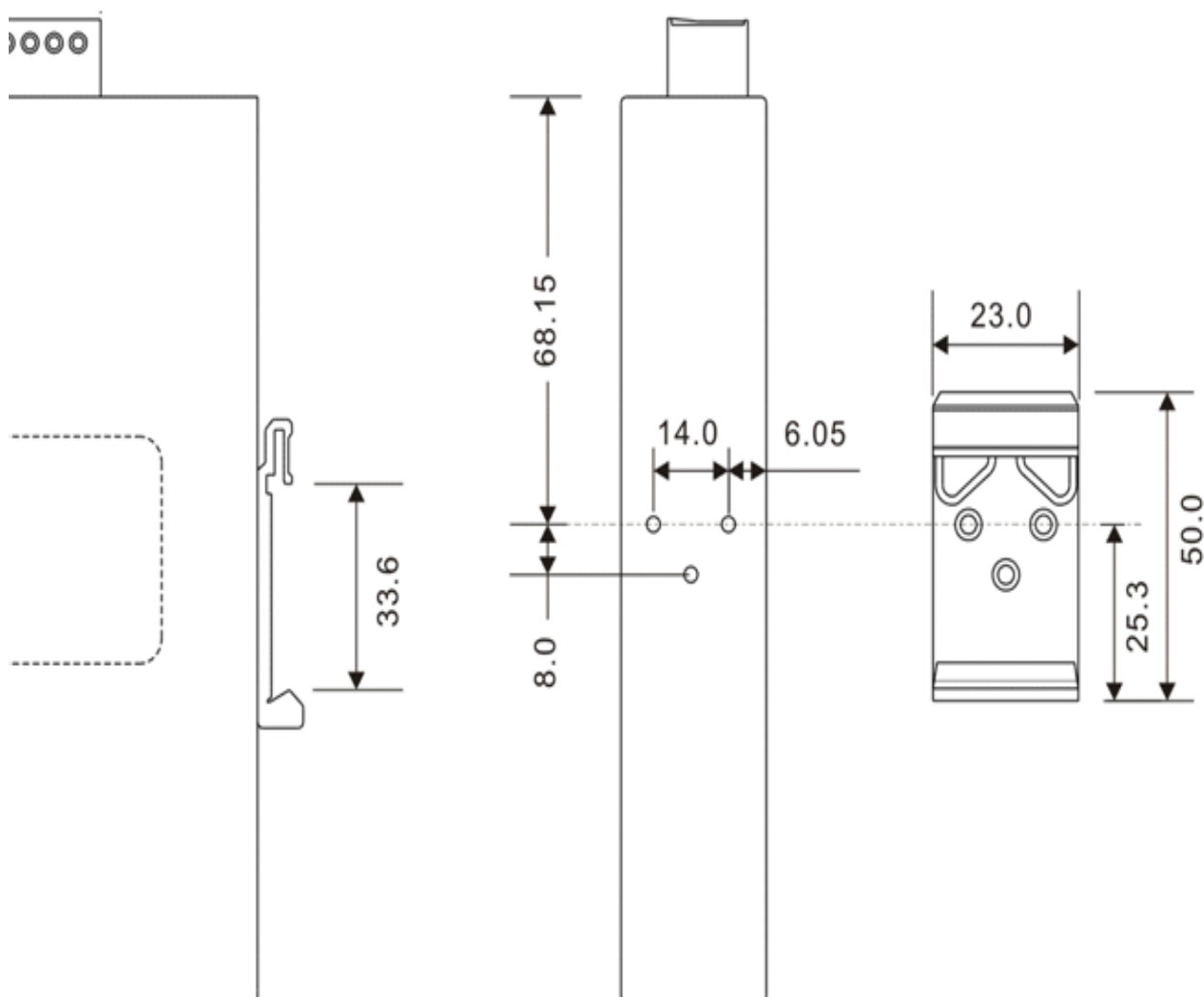
Рис. Размеры DIN-рейки
