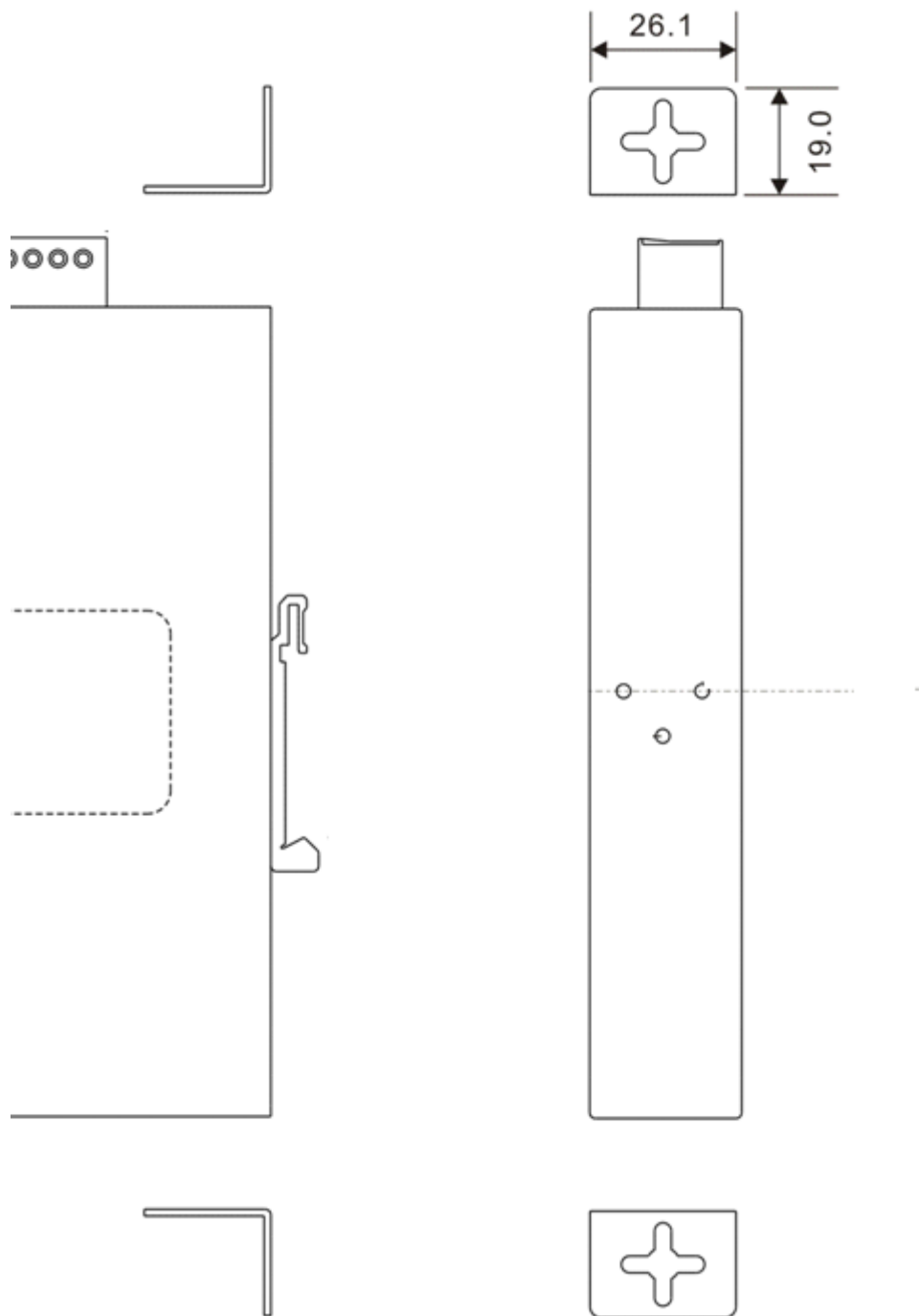
Рис. Размеры настенного крепления
