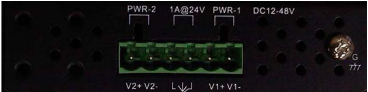
Рис. Подключение питания к SWS-42SFPA-w
